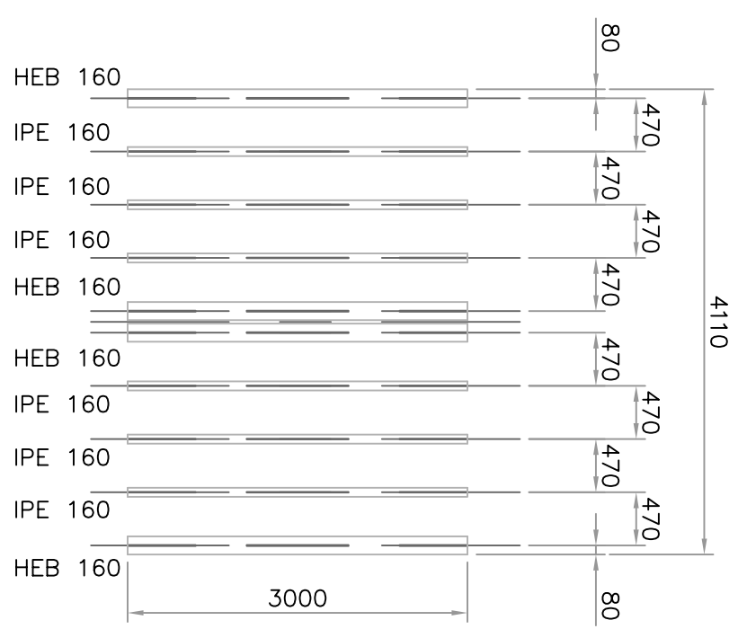
BANCADA A TITULO INFORMATIVO STRUCTURE FOR INFORMATION ESCALA 1:40 SCALE 1:40
